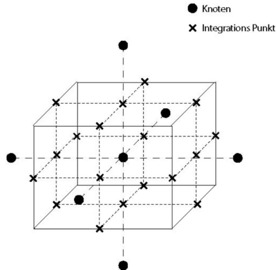
Abbildung 18: Kontrollvolumina, Knoten und Integrationspunkte in der Finite Volumen Methode
