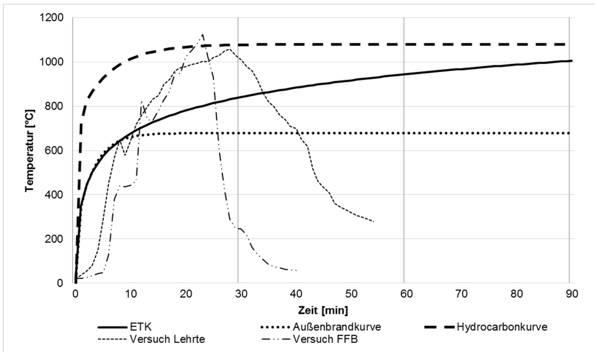
Abbildung 7 Vergleich von Temperaturzeitkurven, Einheitstemperaturzeitkurve (ETK), Außenbrandkurve und Hydrocarbonkurve mit qualitativen Temperaturverläufen (Decke) zweier Realbrandversuche, Brandversuch an der Forschungsstelle für Brandschutztechnik [32] und Versuch aus Versuchsreihe in Lehrte [33]
